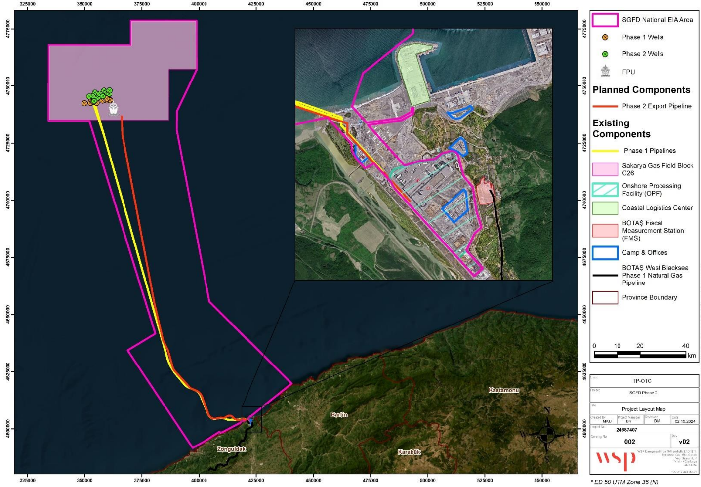
Şekil 11 Proje Yerleşim Planı
